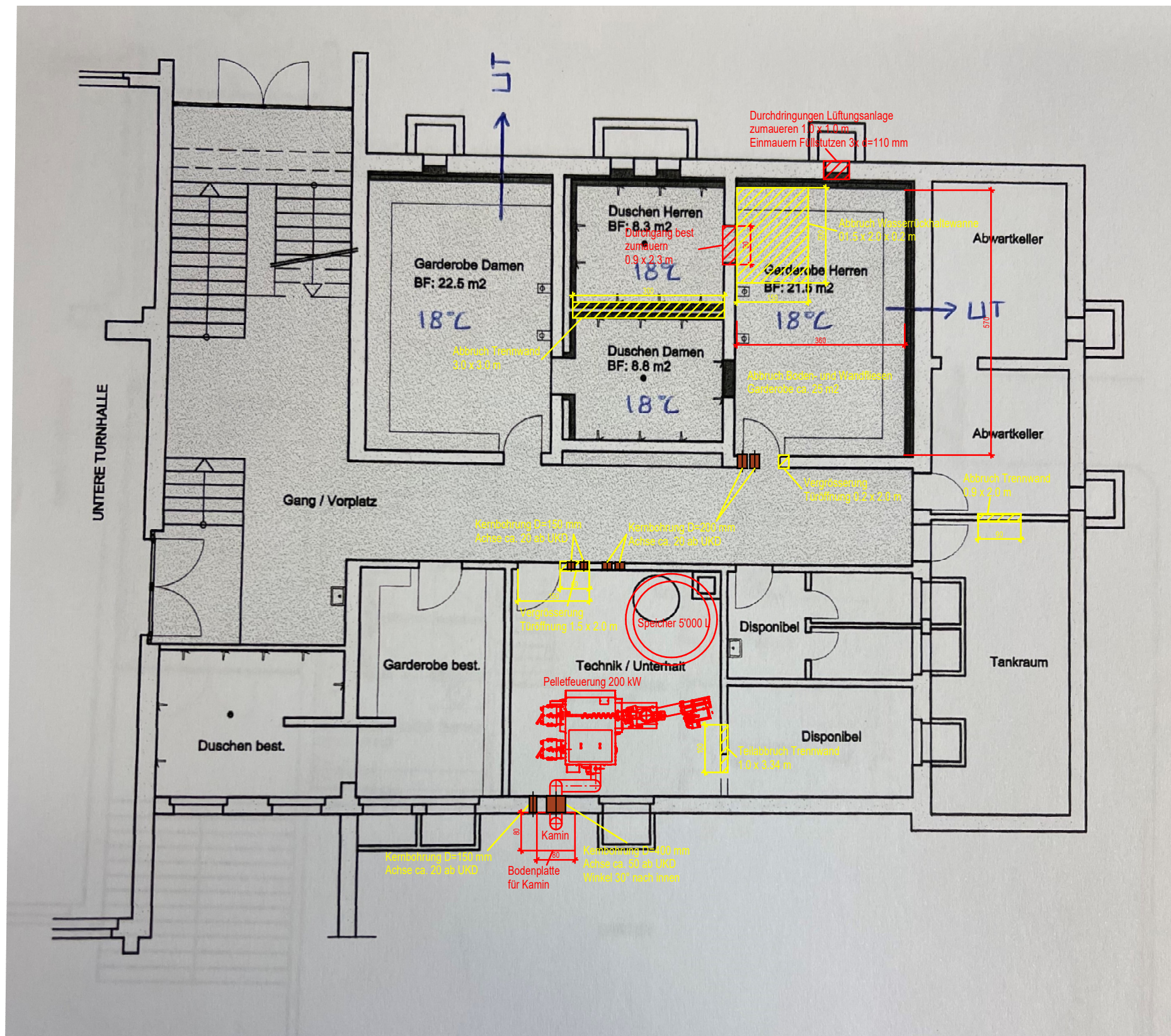
Grundriss
